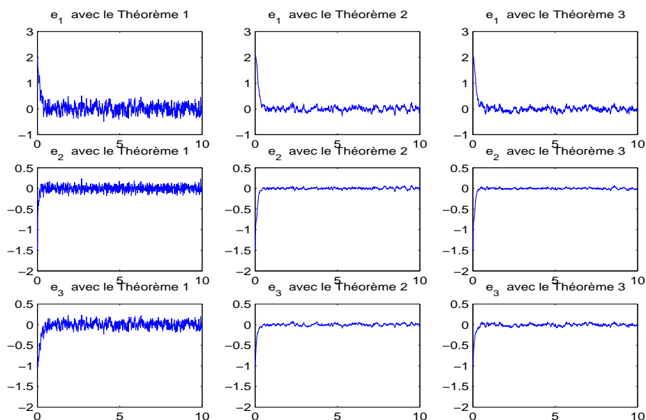
FIG.1. Erreur d'estimation d'état
